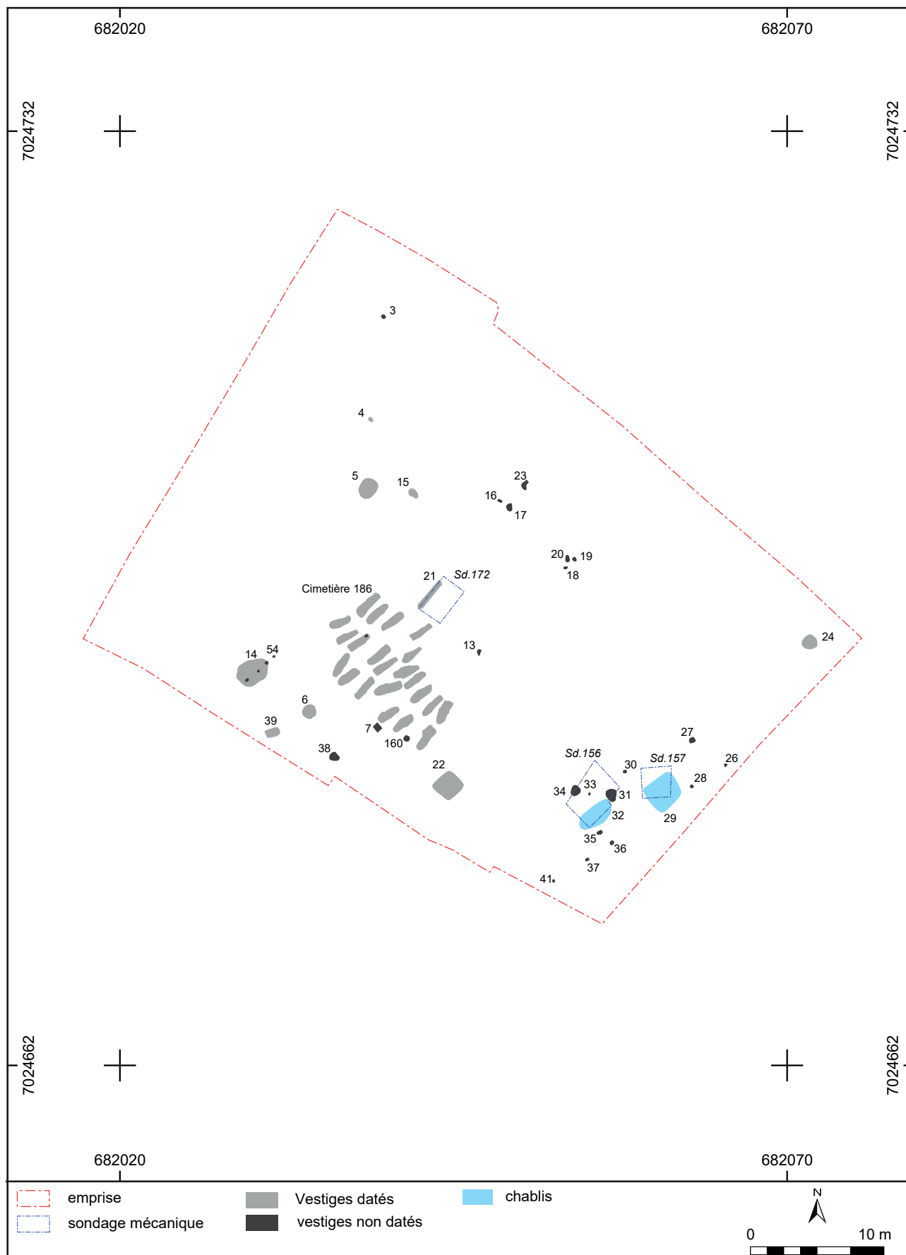
Fig. 64 : Anzin-Saint-Aubin, rue du Maréchal Haig, plan des vestiges non datés, Chr. Costeux - DA62.
