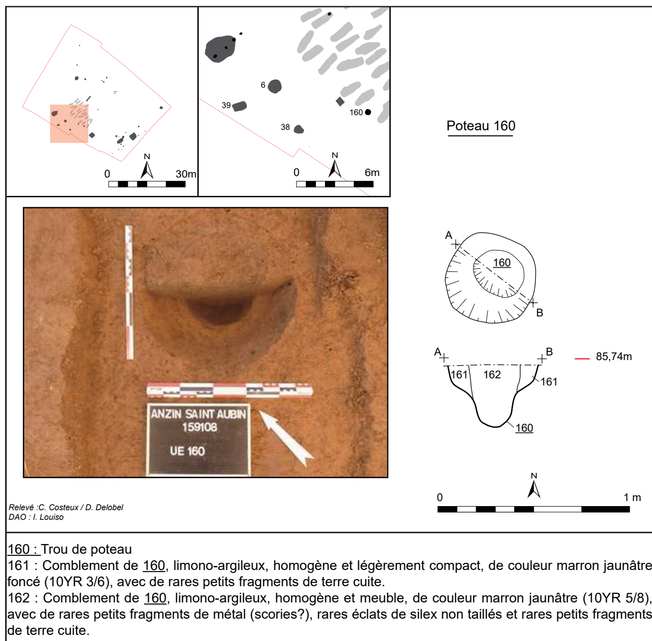
Fig. 66 : Anzin-Saint-Aubin, rue du Maréchal Haig, coupe et plan du poteau UE 160, L. Wilket - DA62.
