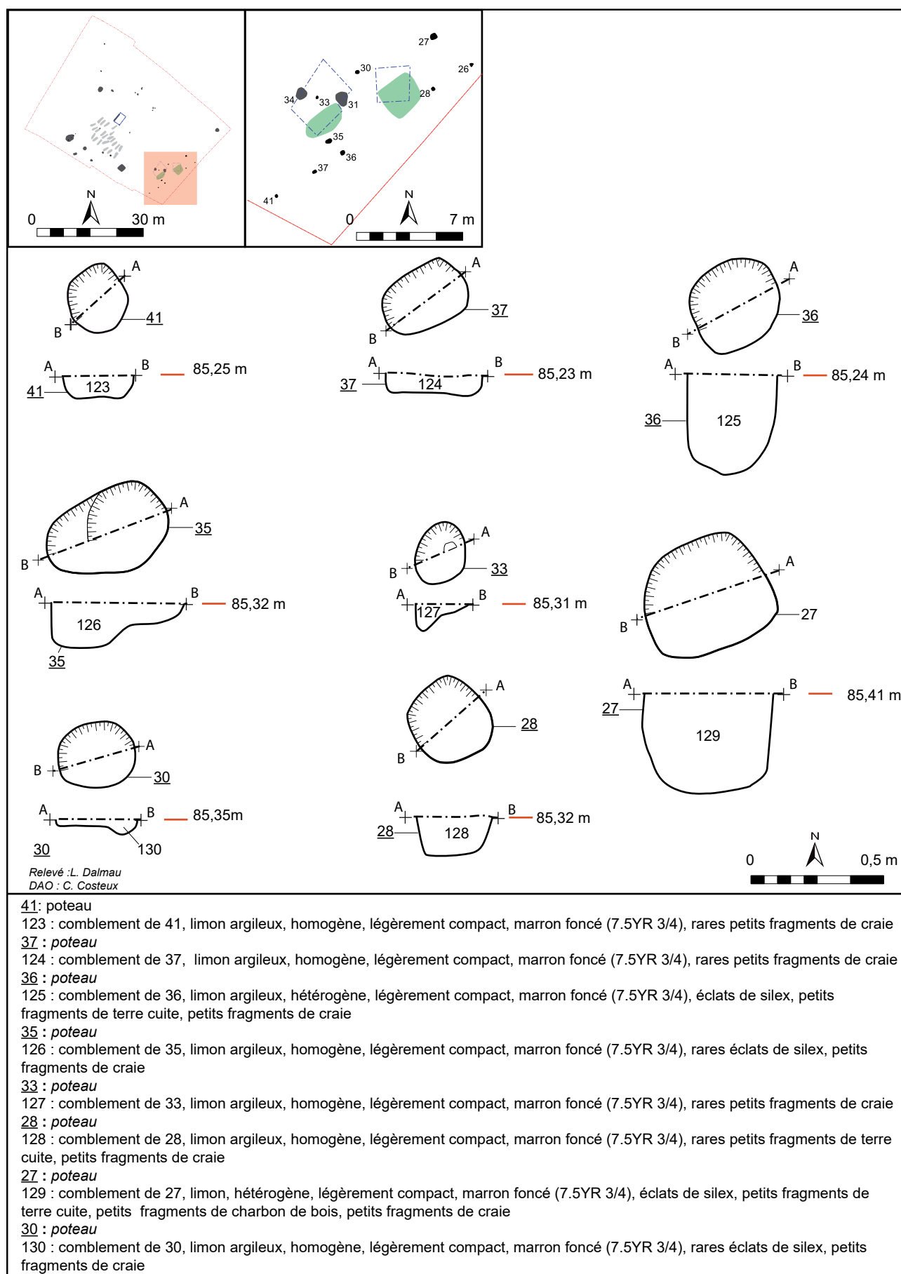
Fig. 69 : Anzin-Saint-Aubin, rue du Maréchal Haig, coupes et plans des structures de la zone sud-est, Chr. Costeux - DA62.
