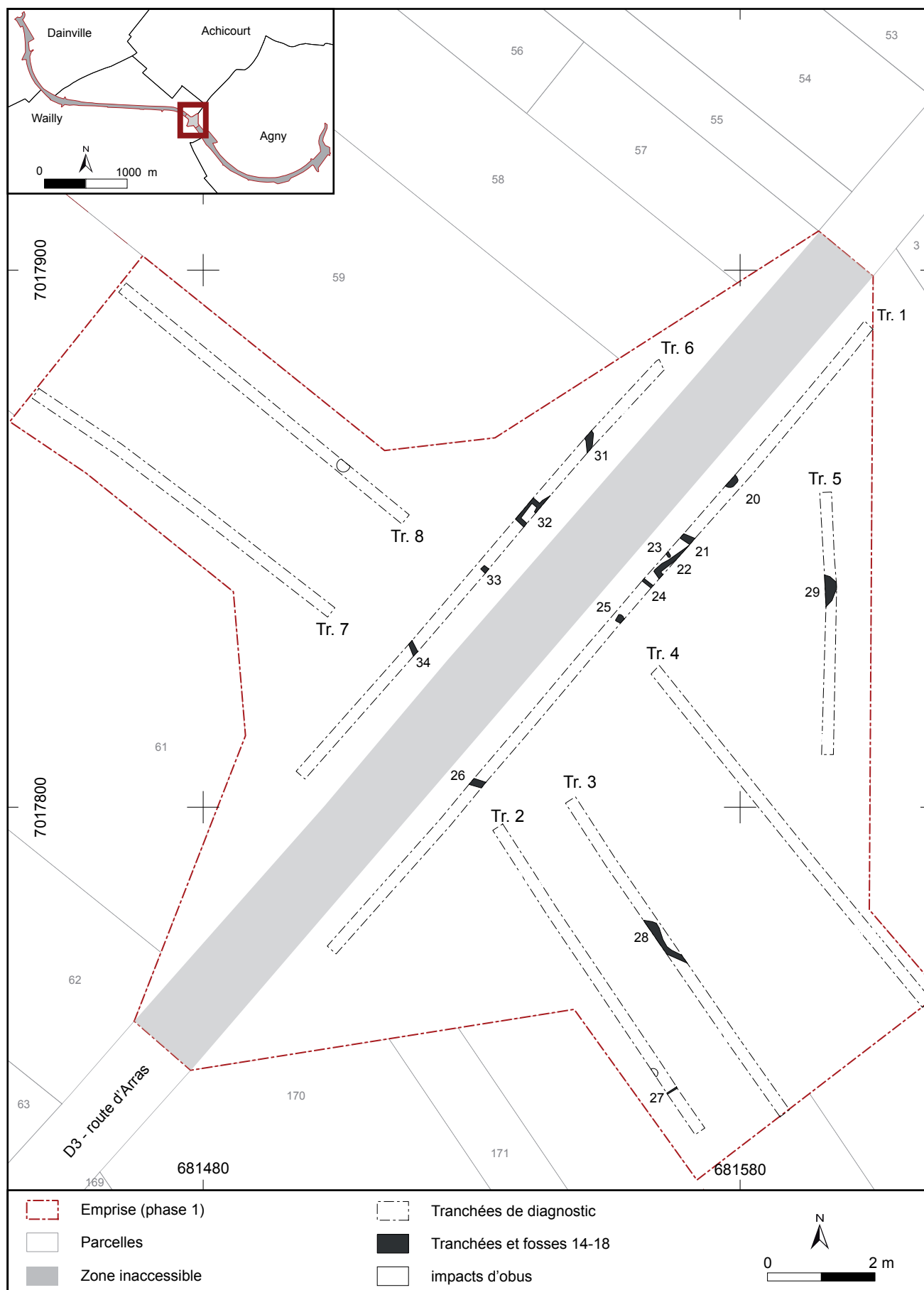
Fig. 7 : RD 60, Giratoire, plan général de l'opération, L. Wilket - DA 62
