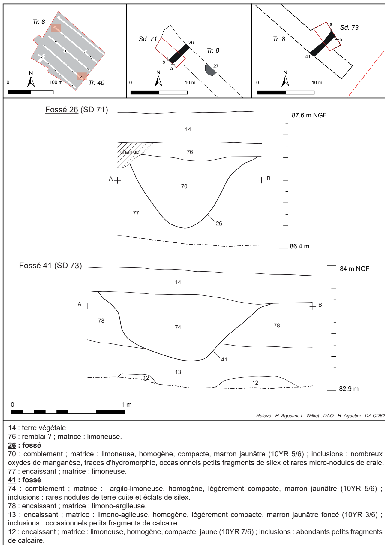
Fig. 29 : Anzin-Saint-Aubin, rue du Maréchal Haig, coupe des fossés 26 et 41, relevé H. Agostini, L. Wilket, DAO H. Agostini - DA, CD 62.
