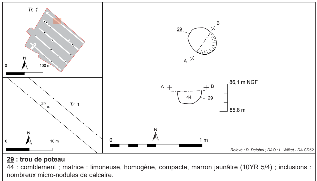
Fig. 33 : Anzin-Saint-Aubin, rue du Maréchal Haig, plan et coupe du trou de poteau 29, relevé D. Delobel, DAO H. Agostini - DA, CD 62.
