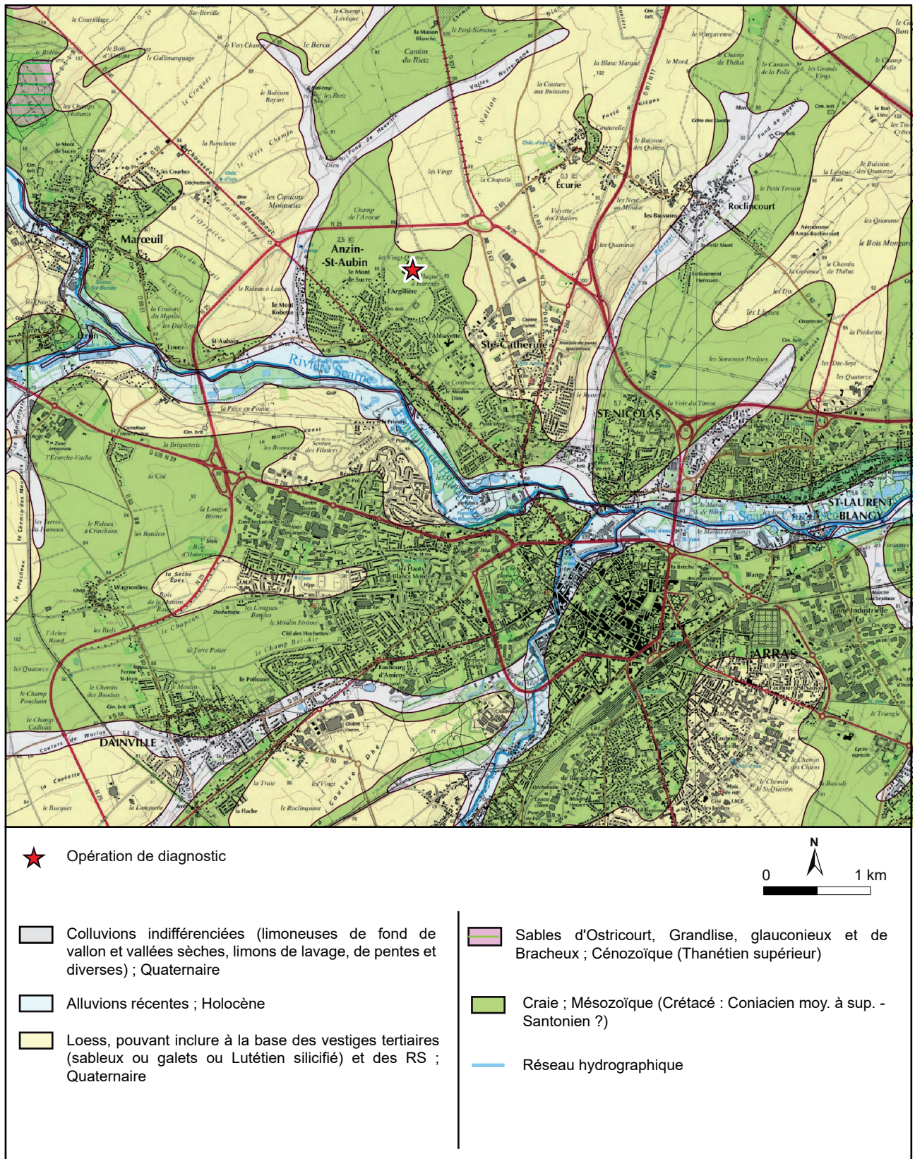
Fig. 7 : Anzin-Saint-Aubin, rue du Maréchal Haig, extrait de la carte géologique au 1/50 000 harmonisée (Lacquement et al. 2004 ; BRGM-Infoterre 2019), M. Meurisse-Fort - DA, CD62.
