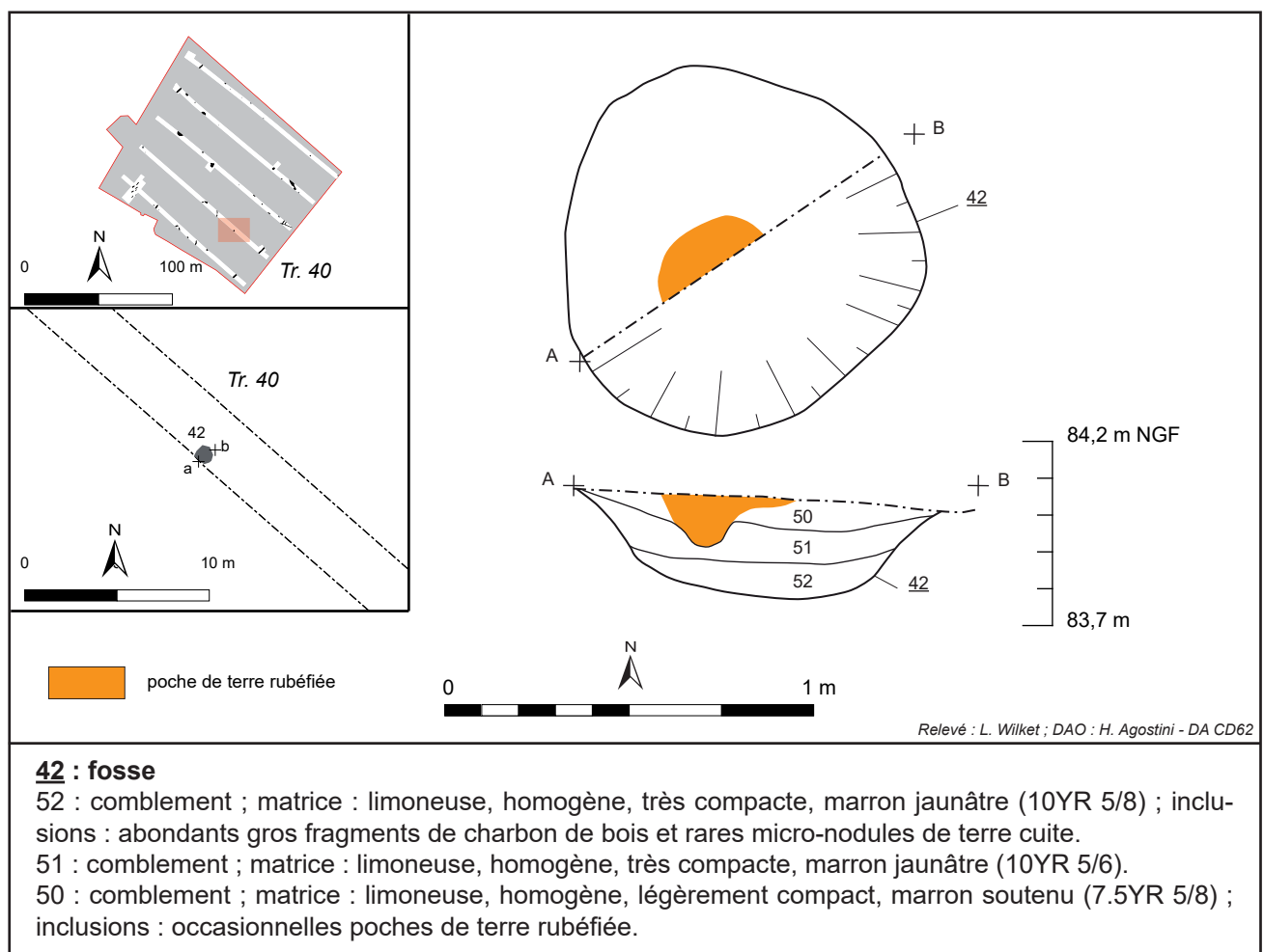
Fig. 30 : Anzin-Saint-Aubin, rue du Maréchal Haig, plan et coupe de la fosse 42, relevé L. Wilket, DAO H. Agostini - DA, CD 62.
