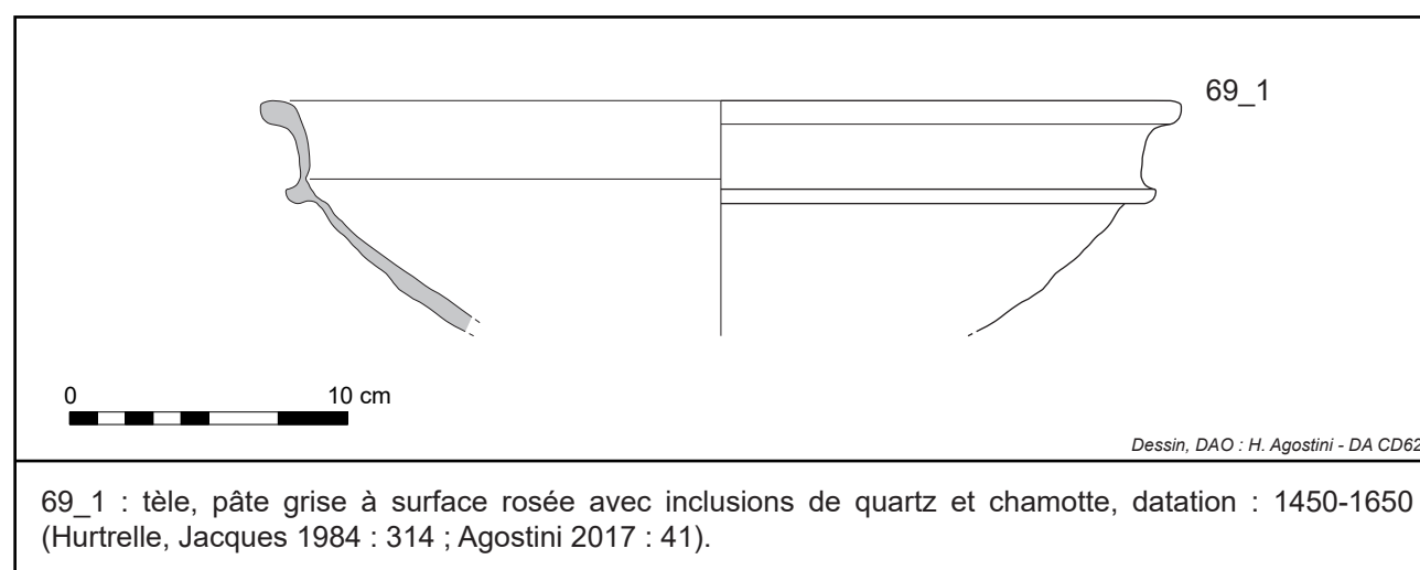
Fig. 21 : Anzin-Saint-Aubin, tèle à lait, dessin/DAO H. Agostini - DA, CD 62.
