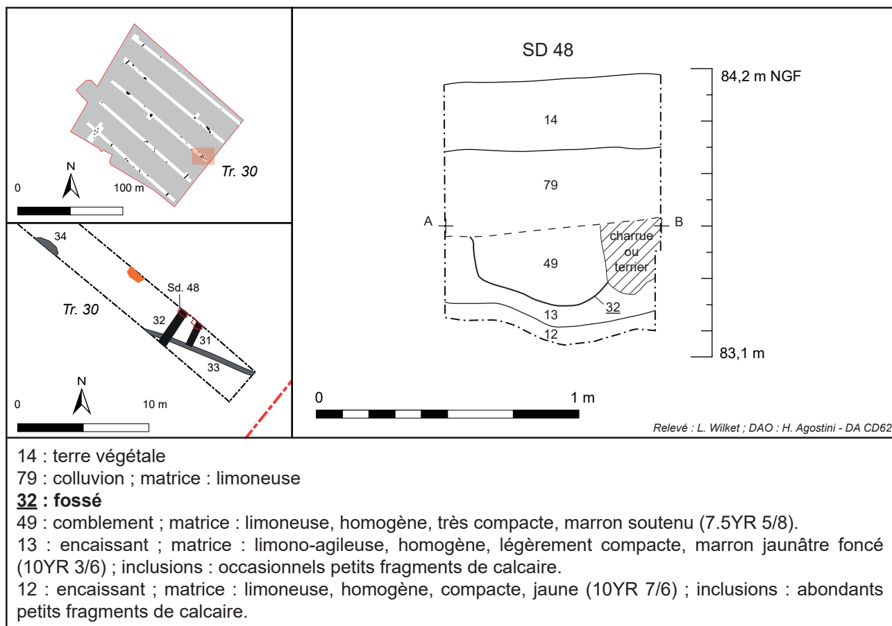
Fig. 13 : Anzin-Saint-Aubin, rue du Maréchal Haig, coupe du fossé 32, relevé L. Wilket, DAO H. Agostini - DA, CD 62.
