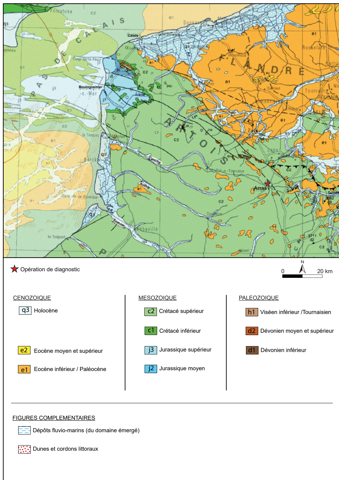
Fig. 6 : Anzin-Saint-Aubin, rue du Maréchal Haig, extrait de la carte géologique au millionième (Chantraine et al. 1996 ; BRGM-Infoterre 2019), M. Meurisse-Fort - DA, CD62.
