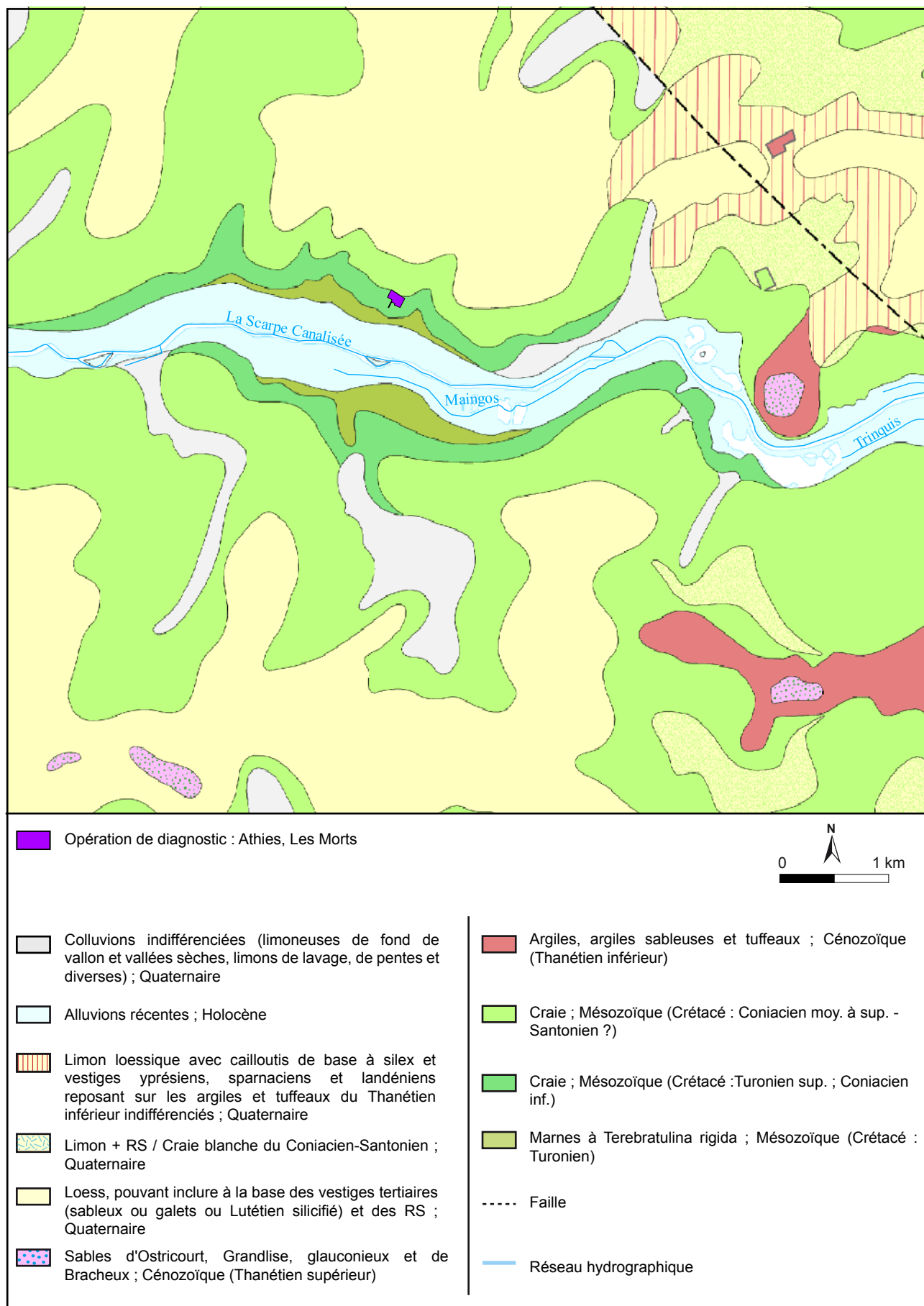
Fig. 6 : Athies, Les Morts, extrait de la carte géologique au 1/50 000 harmonisée (Lacquement et al. 2004; BRGM-Infoterre 2014), M. Meurisse-Fort - CDA CG62.
