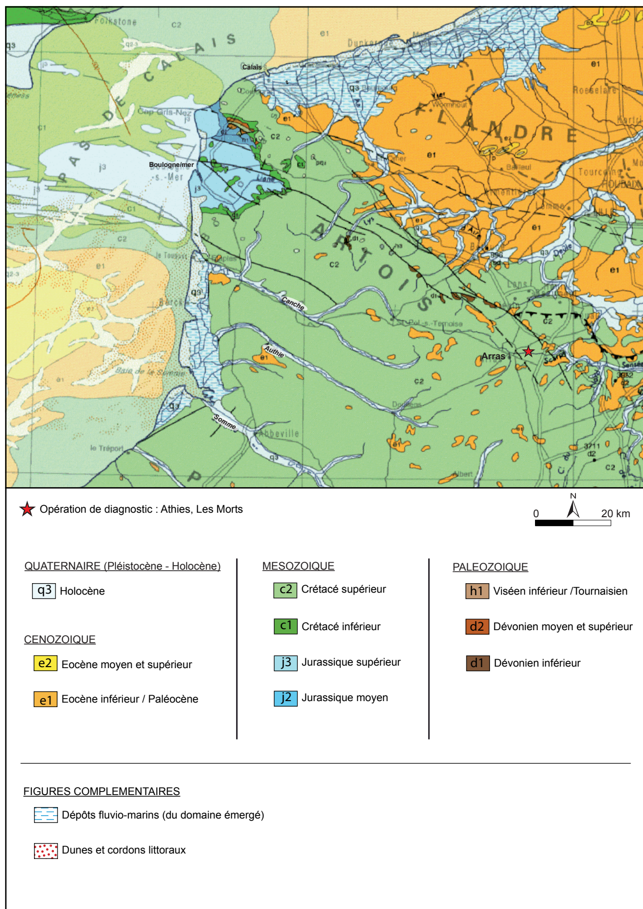
Fig. 5 : Athies, Les Morts, extrait de la carte géologique au millionième (Chantraine et al. 1996; BRGM-Infoterre 2014), M. Meurisse-Fort - CDA CG62
